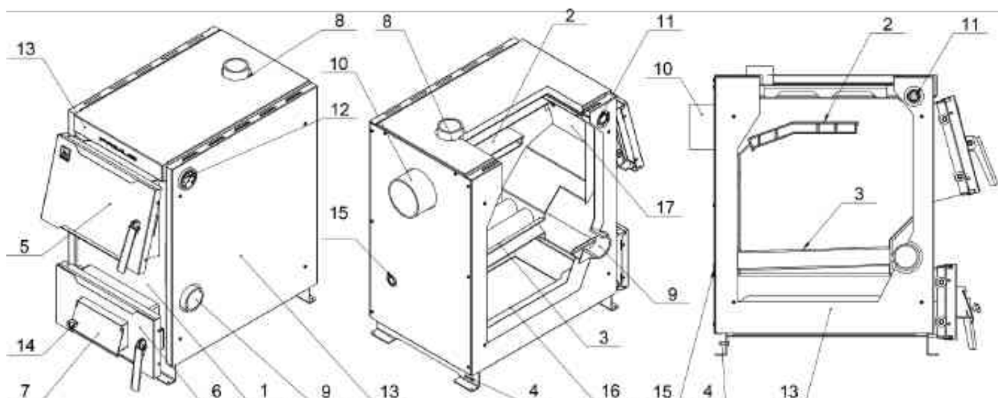
Рис. 1 Устройство котла
